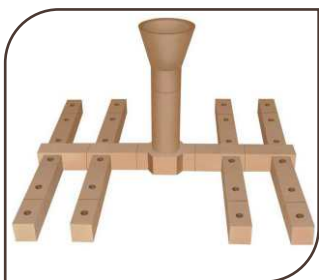
Bottom Pouring Set
